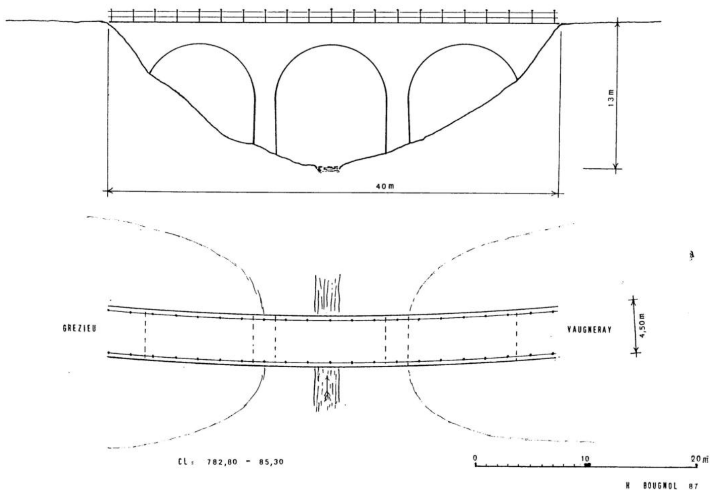
FIG. 9. — Viaduc de la Chaudanne.
