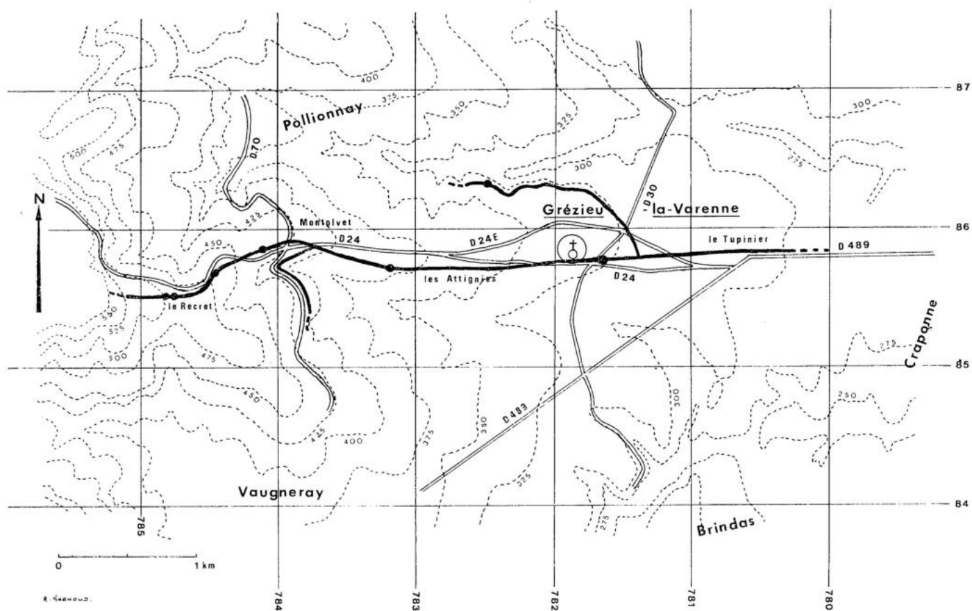
FIG. 6. — Tracé de l'aqueduc de l'Yzeron sur la commune de Grézieu.
