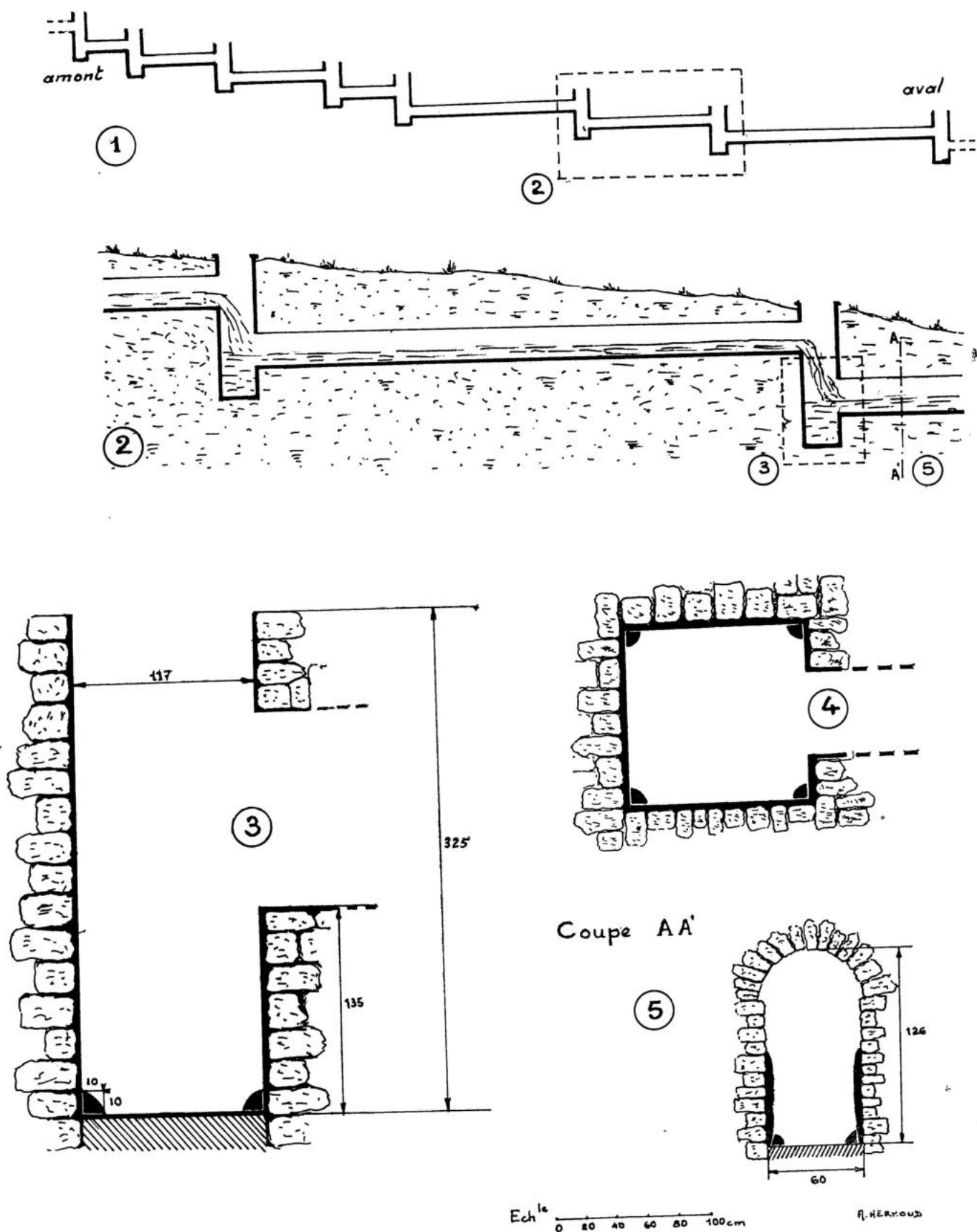
FIG. 7. — Escalier hydraulique de l'aqueduc romain de l'Yzeron.
